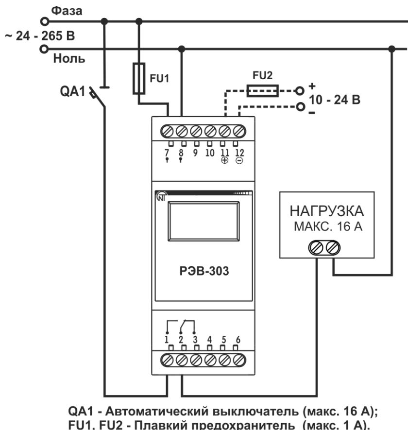
Рисунок 5.1 – Схема подключения РЭВ-303
