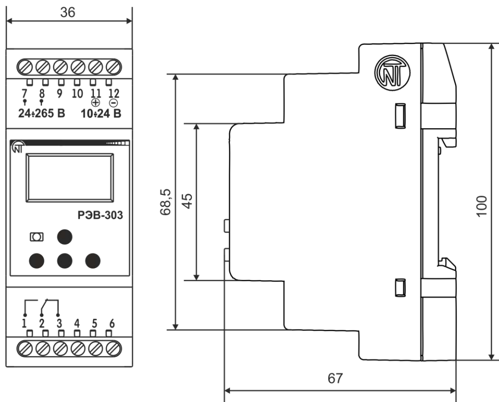
Рисунок 3.1 – Внешний вид и габаритные размеры таймера
